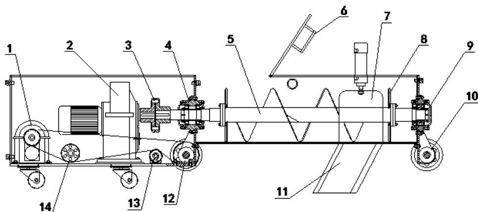
图中：行走电机 1、旋转电机 2、减速器 3、轴承座 4、旋转轴 5、上盖 6、卸料门 7、挡料板 8、定位轴承座 9、后行走轮 10、料斗 11、前行走轮 12、缓冲轮 13、减速轮 14。
